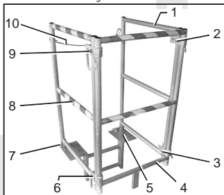
Bild 3 Montage
